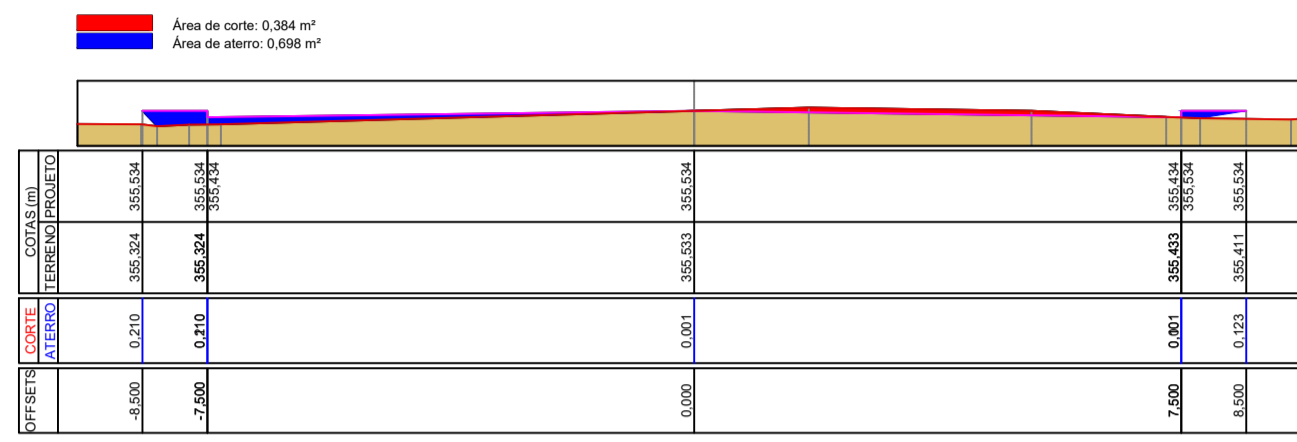
Seção Tipo E10
