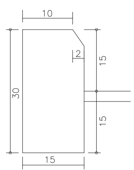
DETALHE - MEIO FIO DETALHAMENTO DE MEIO FIO
