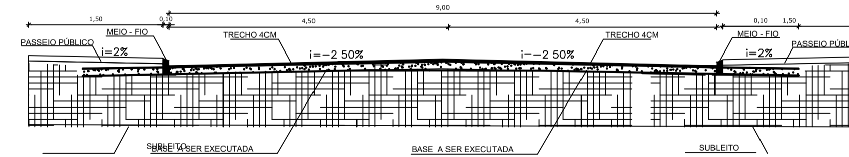
TRECHO - FAIXA ROLAMENTO 4CM CBUQ
