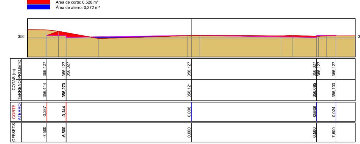
Seção Tipo E13
