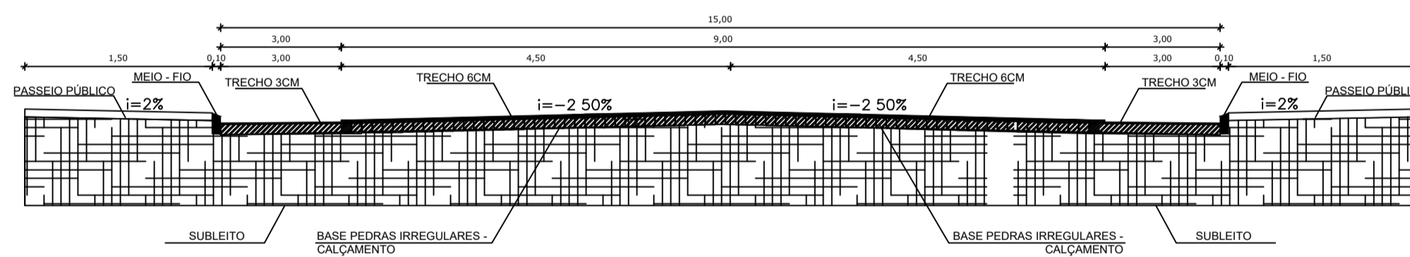
TRECHO - FAIXA 3CM - LARGURA 3M CADA VIA
