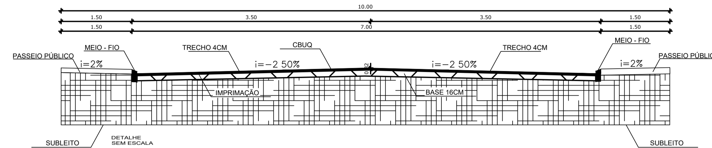
TRECHO - FAIXA ROLAMENTO 4CM CBUQ - LARGURA 3,50M CADA VIA
