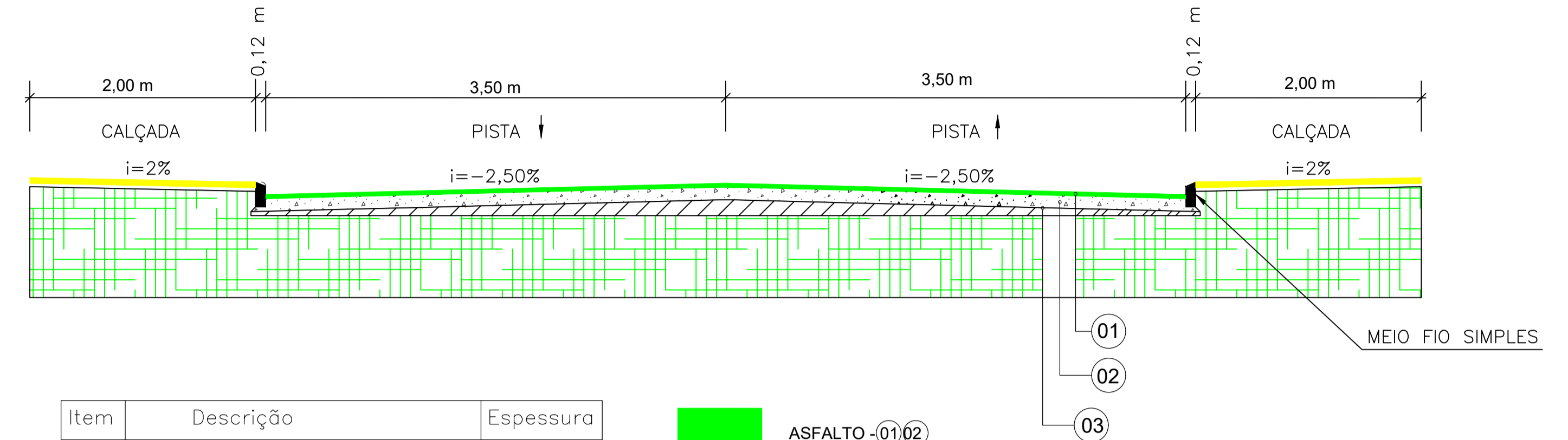
SEÇÃO TIPO DE PAVIMENTAÇÃO
