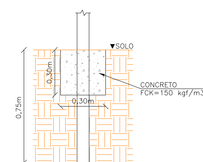
DETALHE DE FIXAÇÃO AO SOLO
