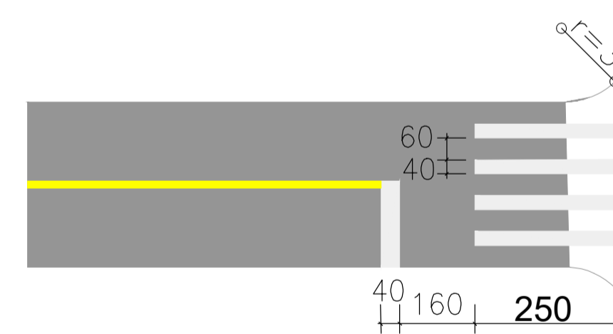
DETALHE FAIXA PEDESTRE
