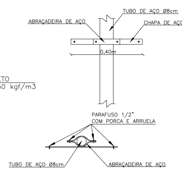
DETALHE DE FIXAÇÃO DO TUBO NA PLACA
