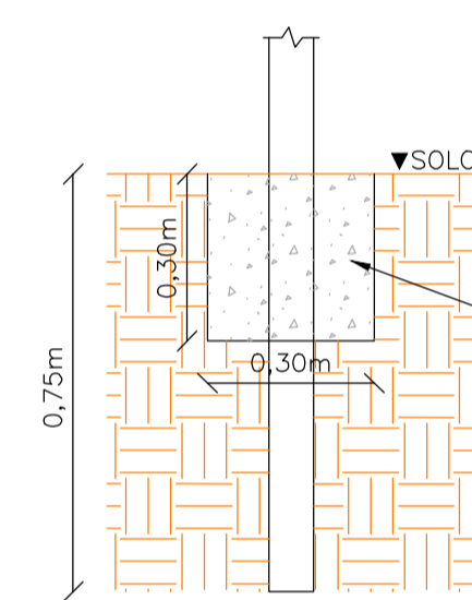
DETALHE DE FIXAÇÃO AO SOLO
